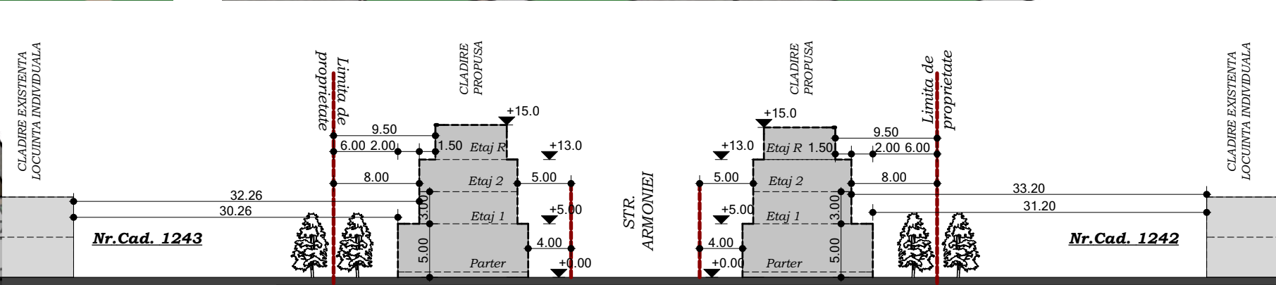
Sectiune caracteristica prin teren
