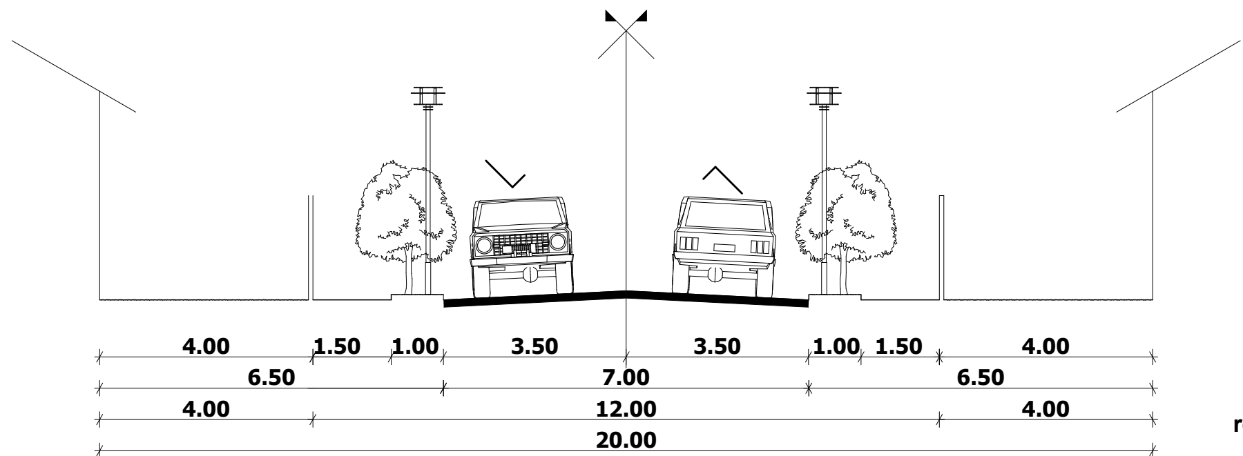
PROFIL TRANSVERSAL DRUM 1-1 SCARA 1:100
