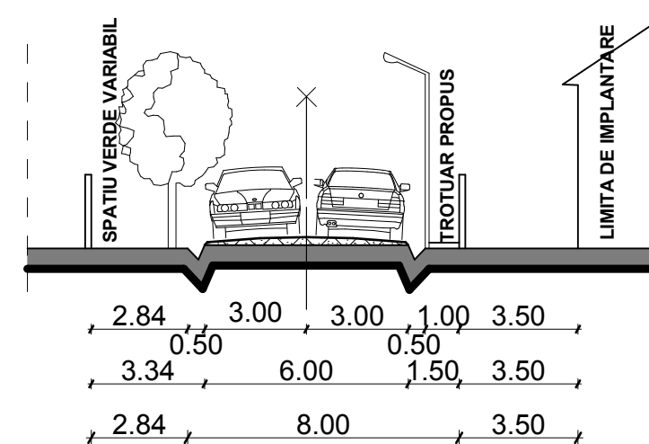
PROFIL TRANSVERSAL B-B - sc. 1:200
