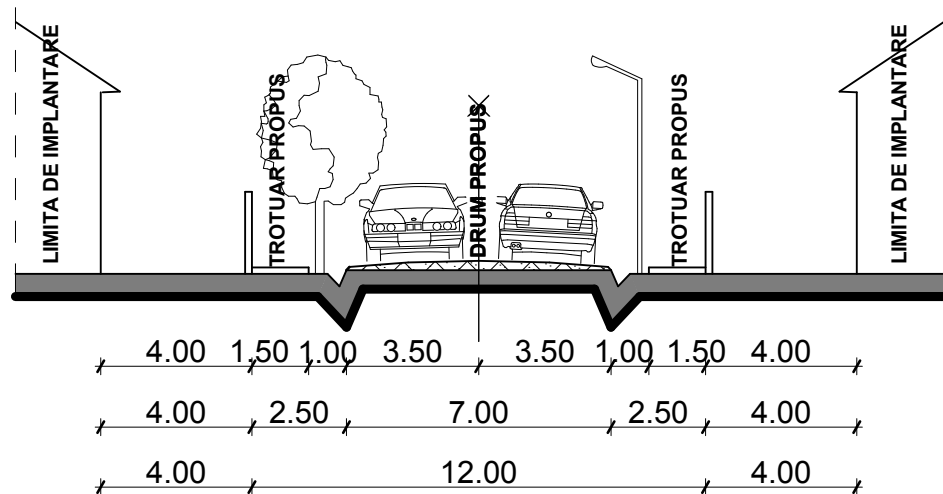
PROFIL TRANSVERSAL A-A - sc. 1:200
