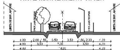
PROFIL TRANSVERSAL A-A - 5C, 1:200
