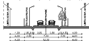
PROFIL TRANSVERSAL B-B - sc. 1:200
