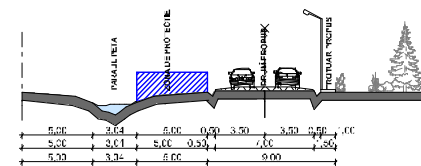
PROFIL TRANSVERSAL C-C - sc. 1:200
