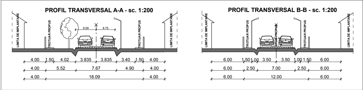
SECTIUNI TRANSVERSALE
