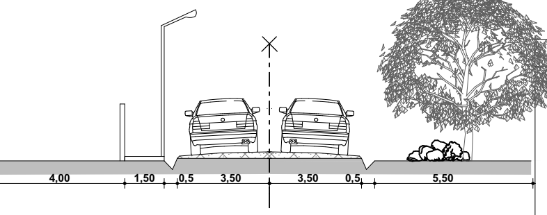
PROFIL STRADAL 9,00 M.+ 6,00 M. SPATIU VERDE
