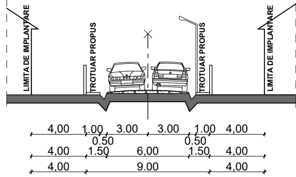
PROFIL TRANSVERSAL B-B - sc. 1:200
