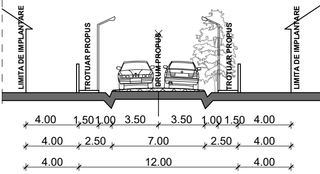
PROFIL TRANSVERSAL A-A - sc. 1:200
